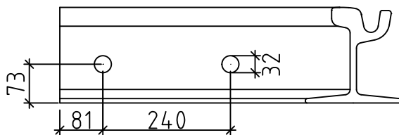
Detalj hållning för skarv järn skala 1:10
